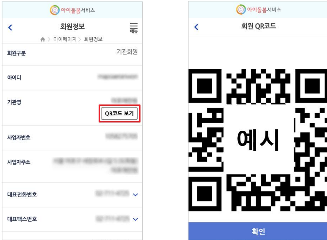
▲모바일웹/모바일앱 화면
